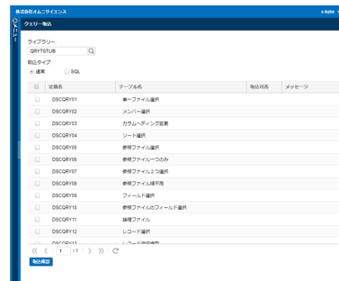
取込定義の選択画面
